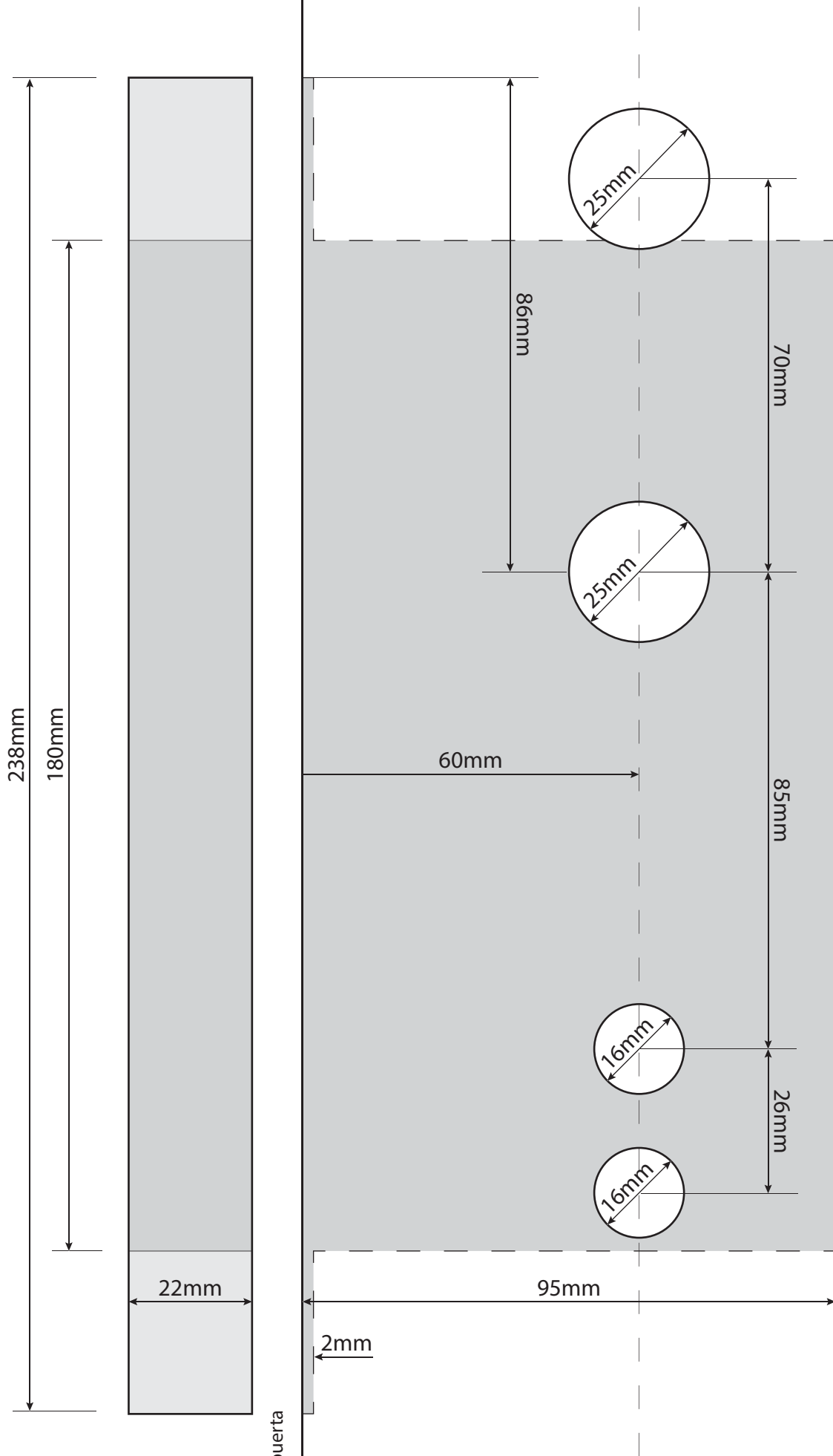
Plantilla de Perforación SHM-F40V/F40/F41
