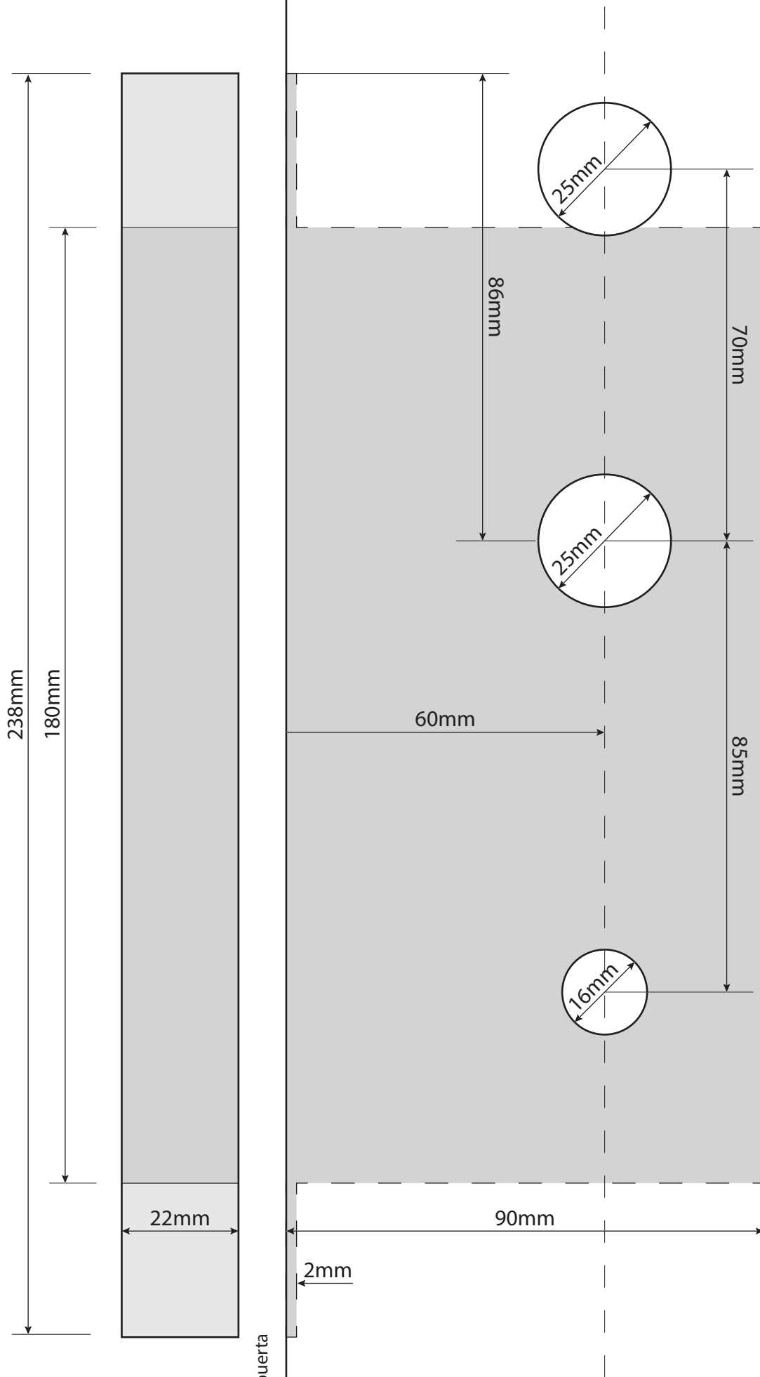
Plantilla de Perforación SHM-H40/50
